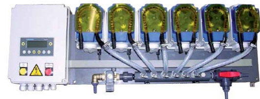
Dosatore elettronico SEKO con centralina. I dosatori sono fino a sette pompe di dosaggio.
