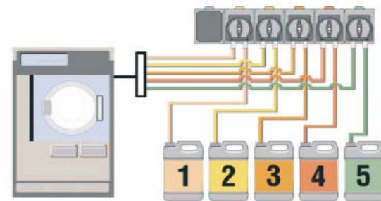
Schema del sistema di lavaggio automatico
